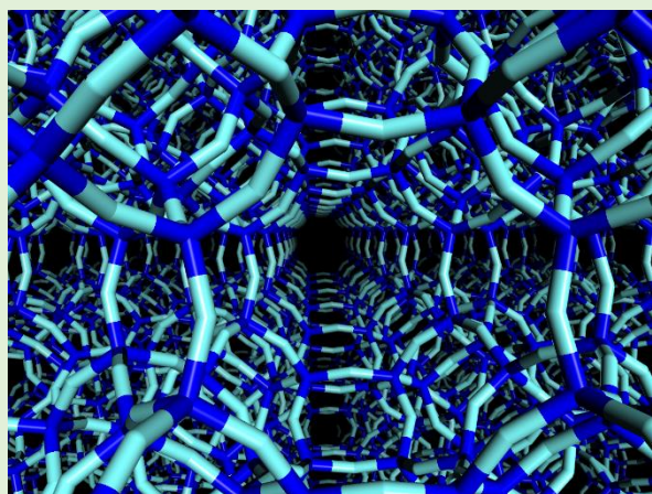
ITQで中村が合成に挑んだ RUB-13ゼオライトの結晶構造モデル
